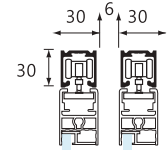
緩衝懸吊鋁門側剖圖
