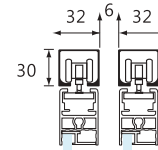
一般懸吊鋁門側剖圖
