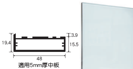
鏡面A型-無背板
