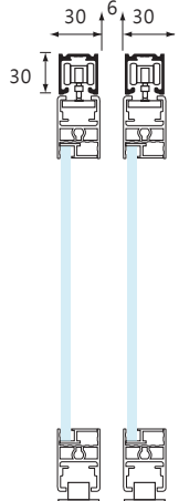
緩衝懸吊鋁門側剖圖
