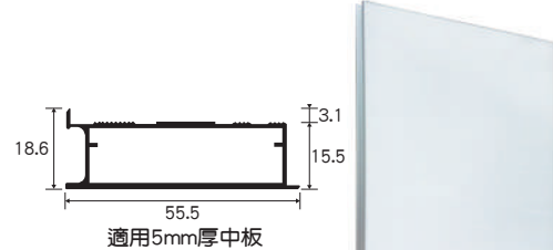
鏡面U型-有背板
