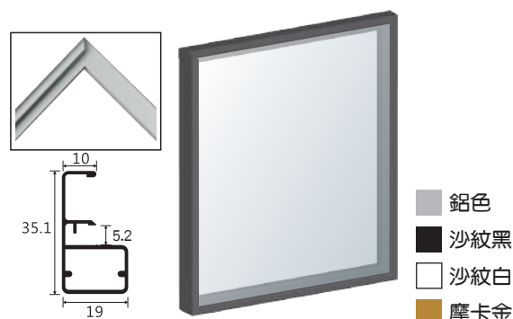
A-1AF 細鋁框【有把手】
