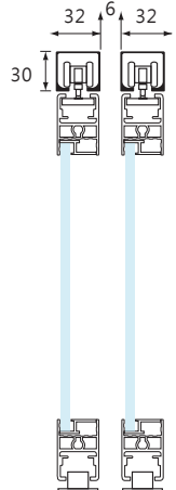
一般懸吊鋁門側剖圖
