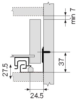
軌道安裝空間需求
