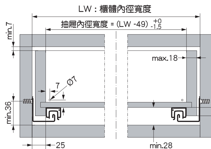
抽屜組裝位置圖
