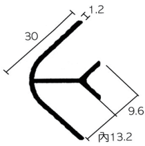
鋁轉角條
