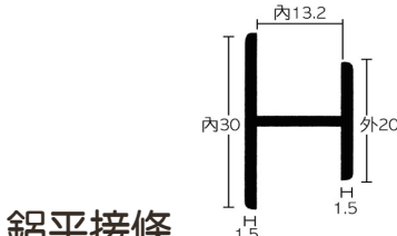
鋁平接條
