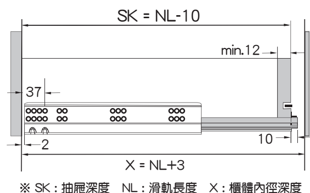
外抽尺寸圖
