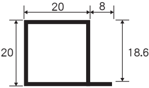
D型-層板鋁條
