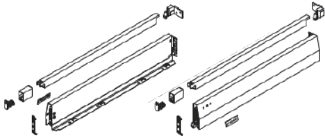
高抽組含邊桿-164
