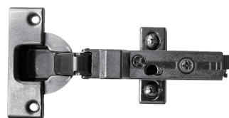
110°緩衝鉸鍊-3分
