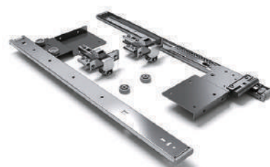
掀板滑軌【載重:20kg】
